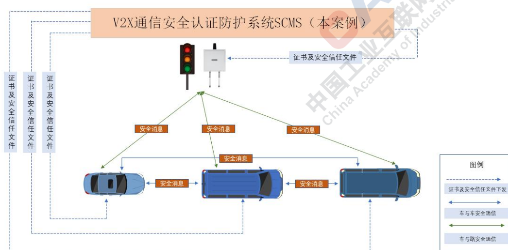
图 3.4 SCMS 系统应用架构图
