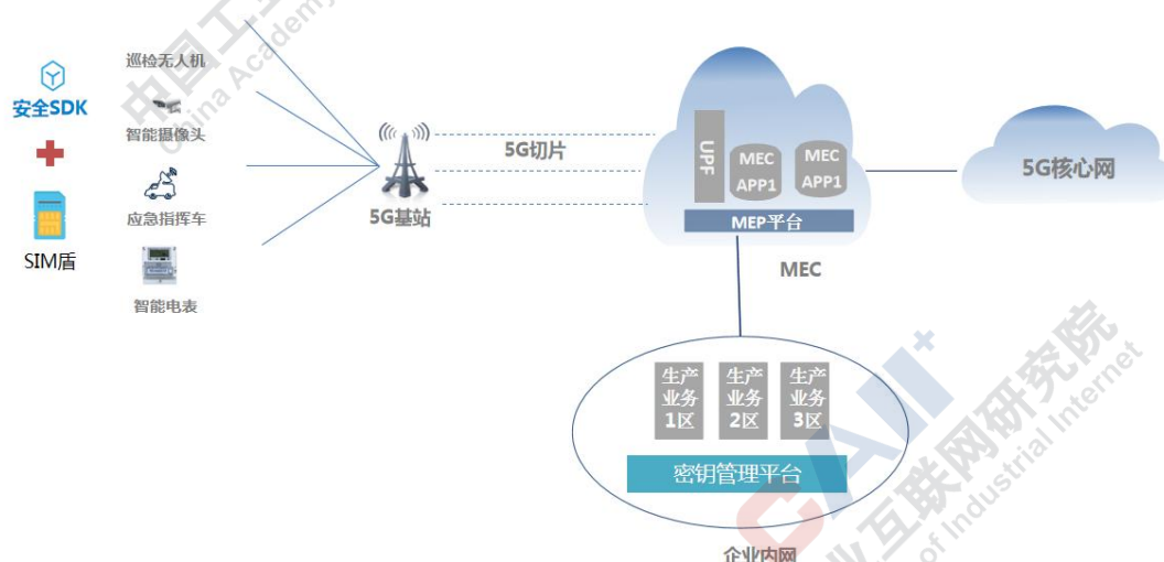
图 7.1 总体技术架构图
