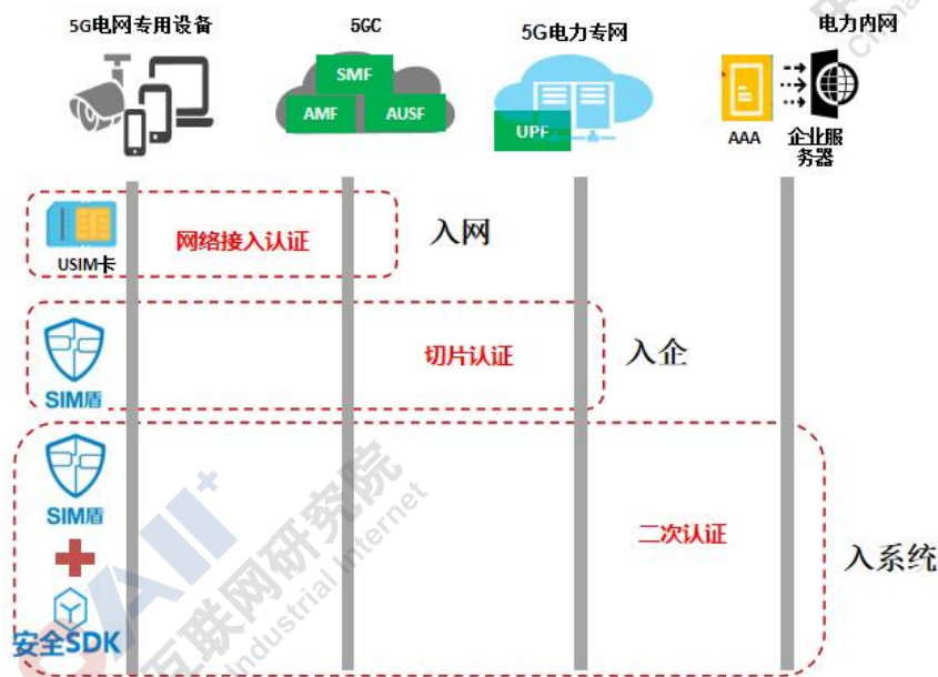
图 7.2 SIM 盾认证机制
