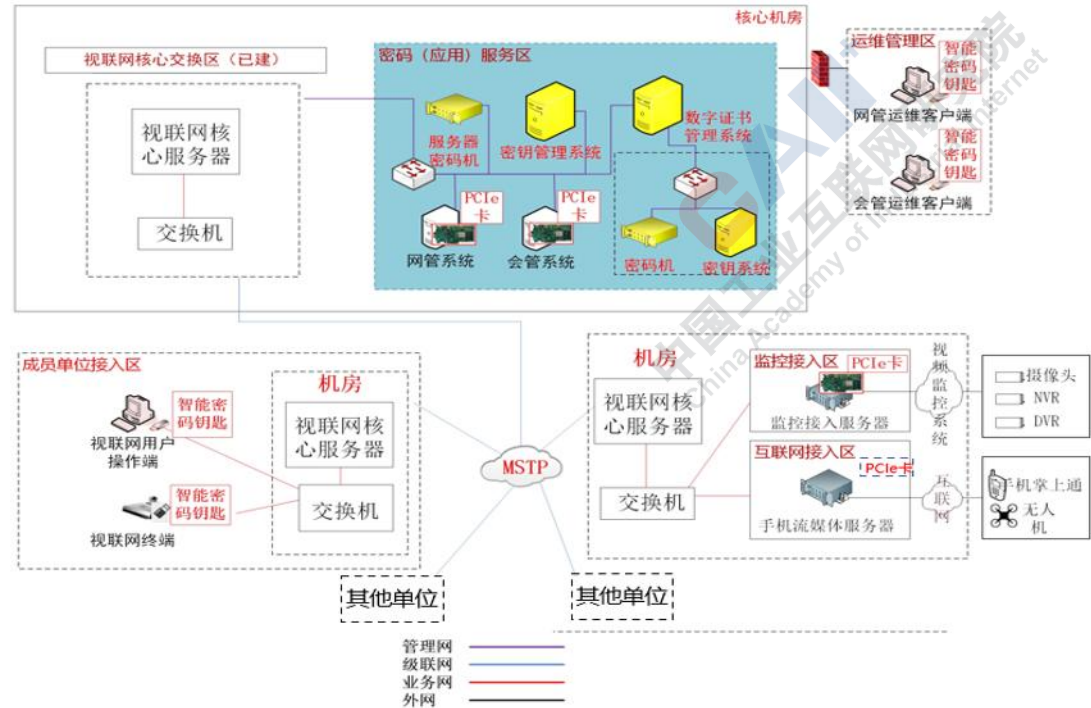
图 5.2 某省国密升级改造设备部署图
