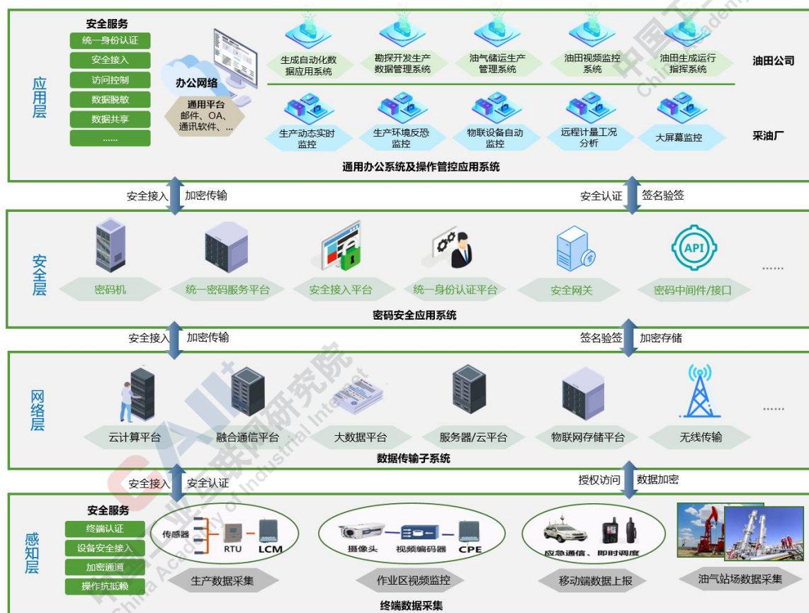
图 8.2 石油工控系统密码应用架构
