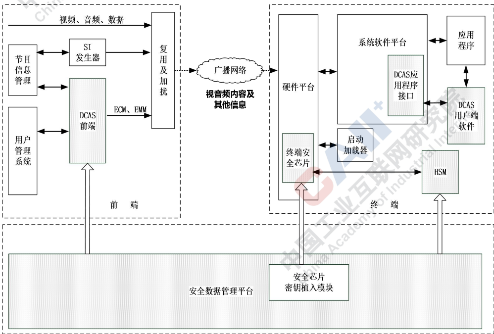
图 14.1 DCAS 系统架构图
