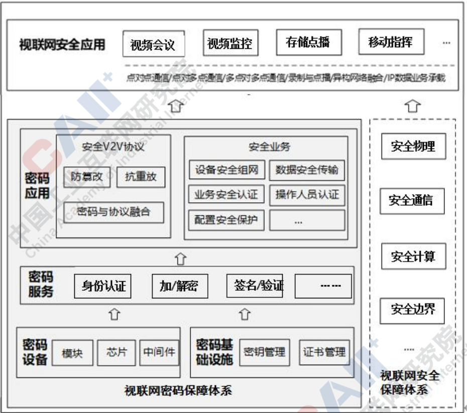
图 5.1 电子政务视联网密码应用总体框架
